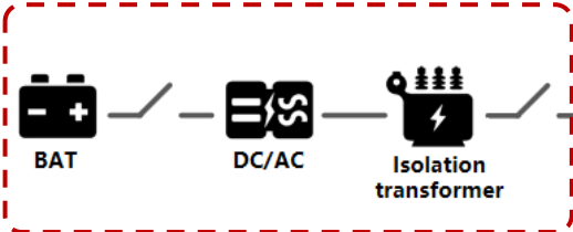
Топологічна схема
