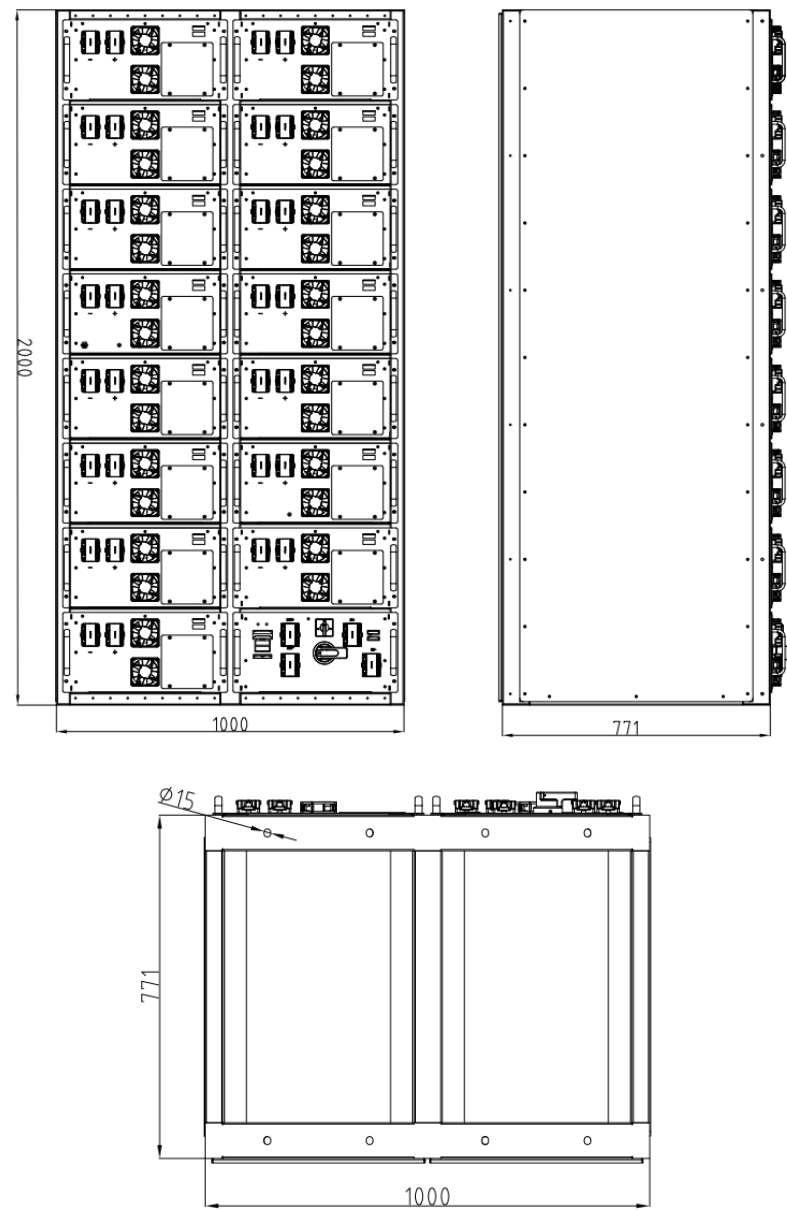
EBC-768V/314Ah-LFP-ABMS
